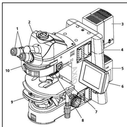
Рисунок 2 – Общий вид моторизованной модели микроскопа Axio Imager
