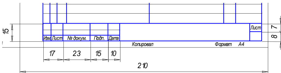
Рисунок 13.4 - Основная надпись для спецификации (последующие листы)
