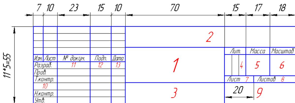
Рисунок 13.2 - Основная надпись
