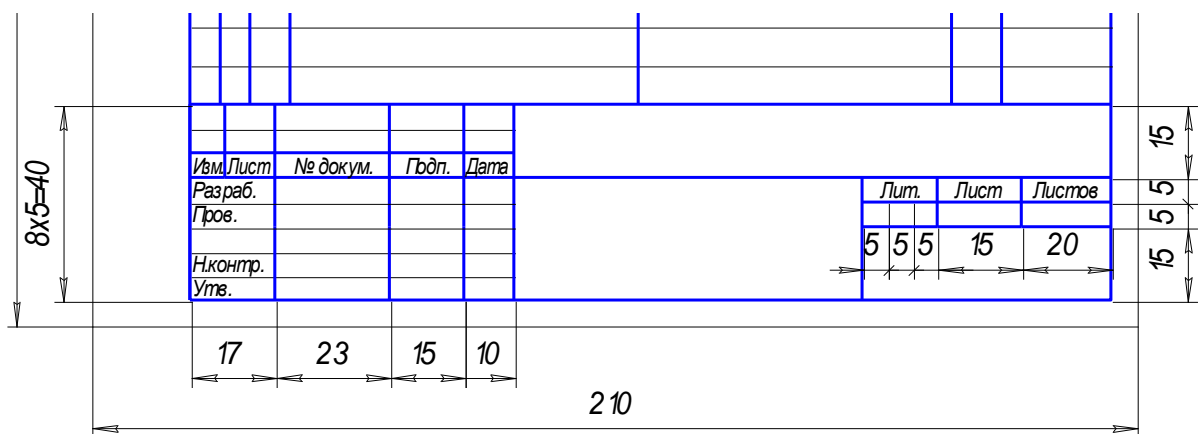
Рисунок 13.3 - Основная надпись для спецификаций (первый лист)
